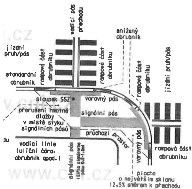
Vzor č. 1 - řešení u výjezdu z parkoviště
