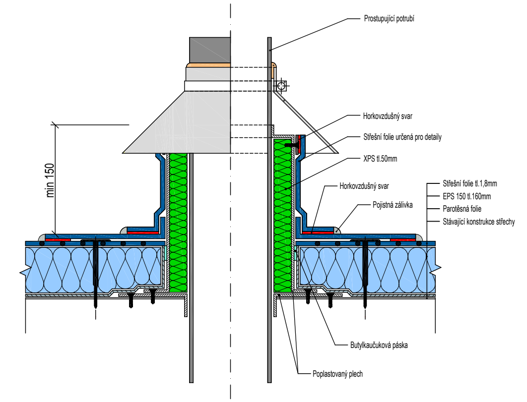
Opravení prostupu potrubí se zateplením
