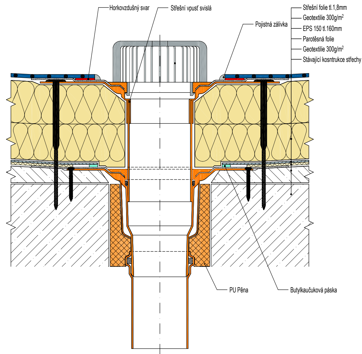
Napojení fólie FATRAFOL na dvoustupňový střešní vtok
