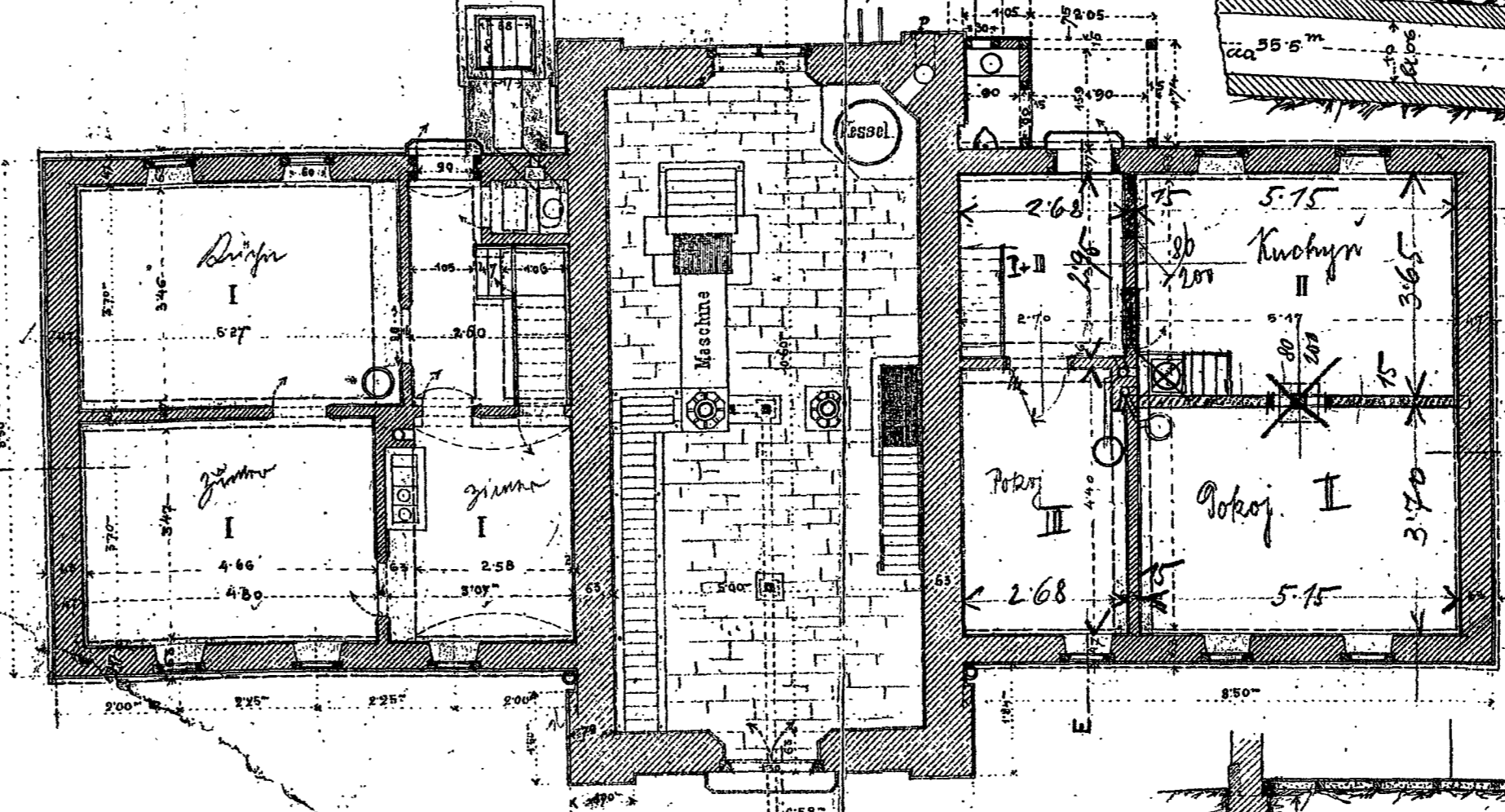
Grundriss vom Erdgeschoss
