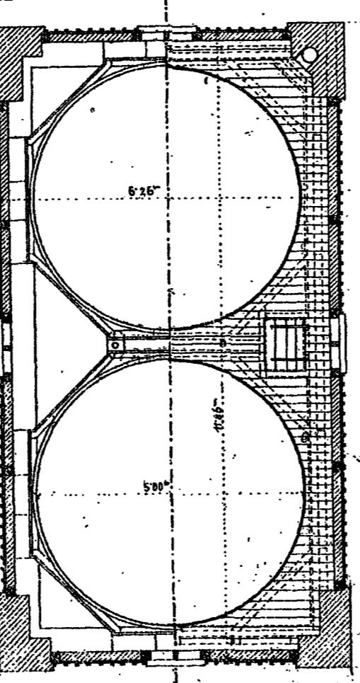
Grundriss über den Trägern
